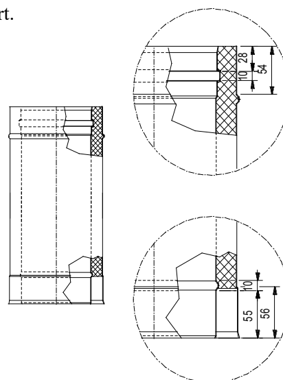
Bild 3: Längenelement
