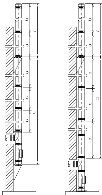
Bild 1: Aufbauhöhen
