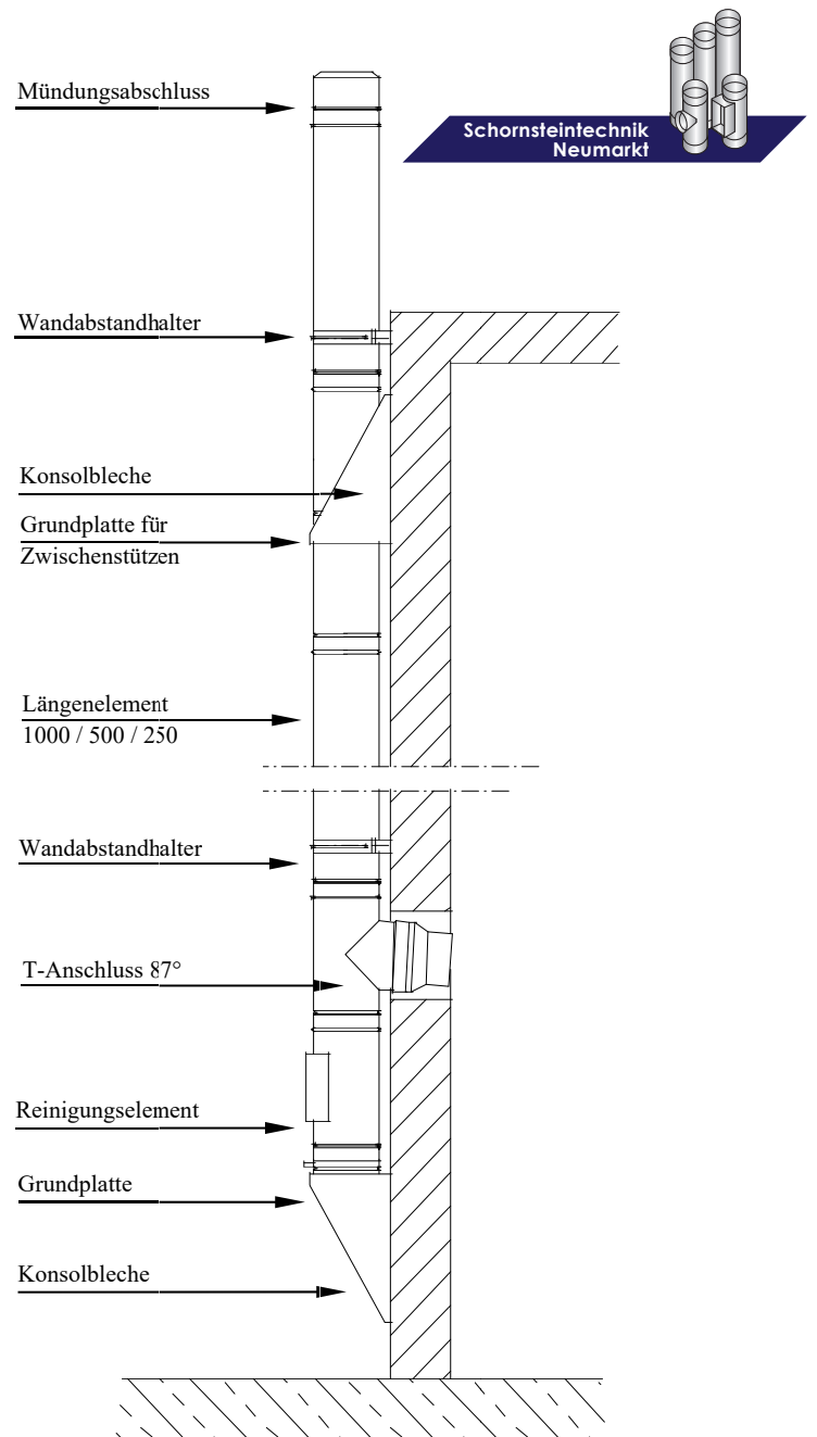
Bild 9: Aufbau mit Zwischenstütze
