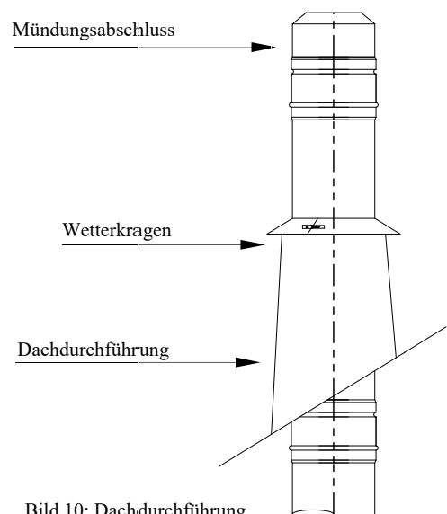
Bild 10: Dachdurchführung
