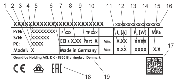
Abb. 18 Beispielhaftes Typenschild
