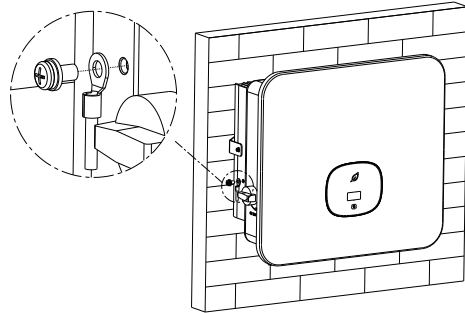
Abb. 6.1 Erdungsschema
