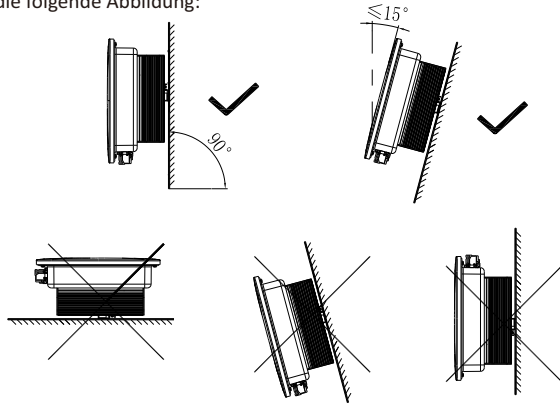
Abb. 5.1 Installationschema
